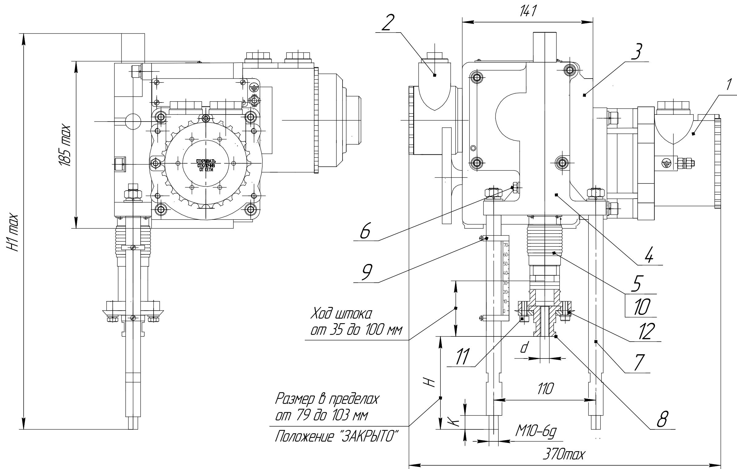
Рисунок А.1 – Общий вид габаритные и присоединительные размеры МЭПК6300-ИСТ4
