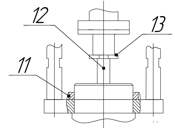
Рисунок А.3 – Схема установки механизма на арматуре
