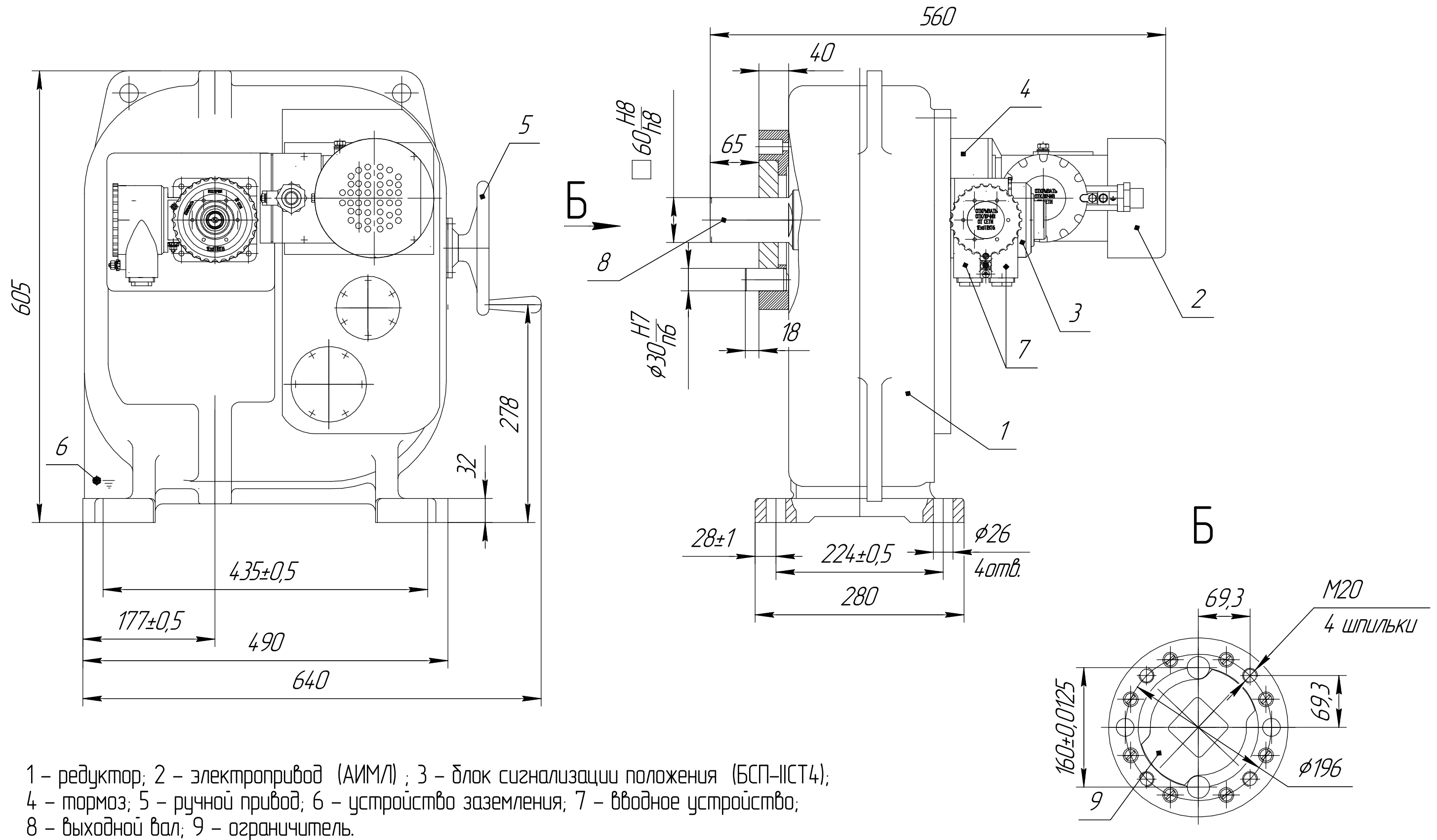
Рисунок А.2 – Общий вид, габаритные и присоединительные размеры механизма МЭОФ-ІВТ4 группы 4000
