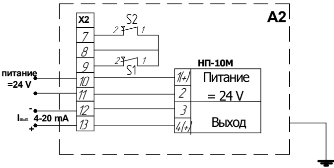
Рисунок Б.2 - Схема электрическая с блоком БСПТ-ИСТ4 Остальное см. рисунок Б.1
