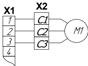
Рисунок Б.2–Схема механизма трехфазного исполнения Остальное см. рис. Б.1
