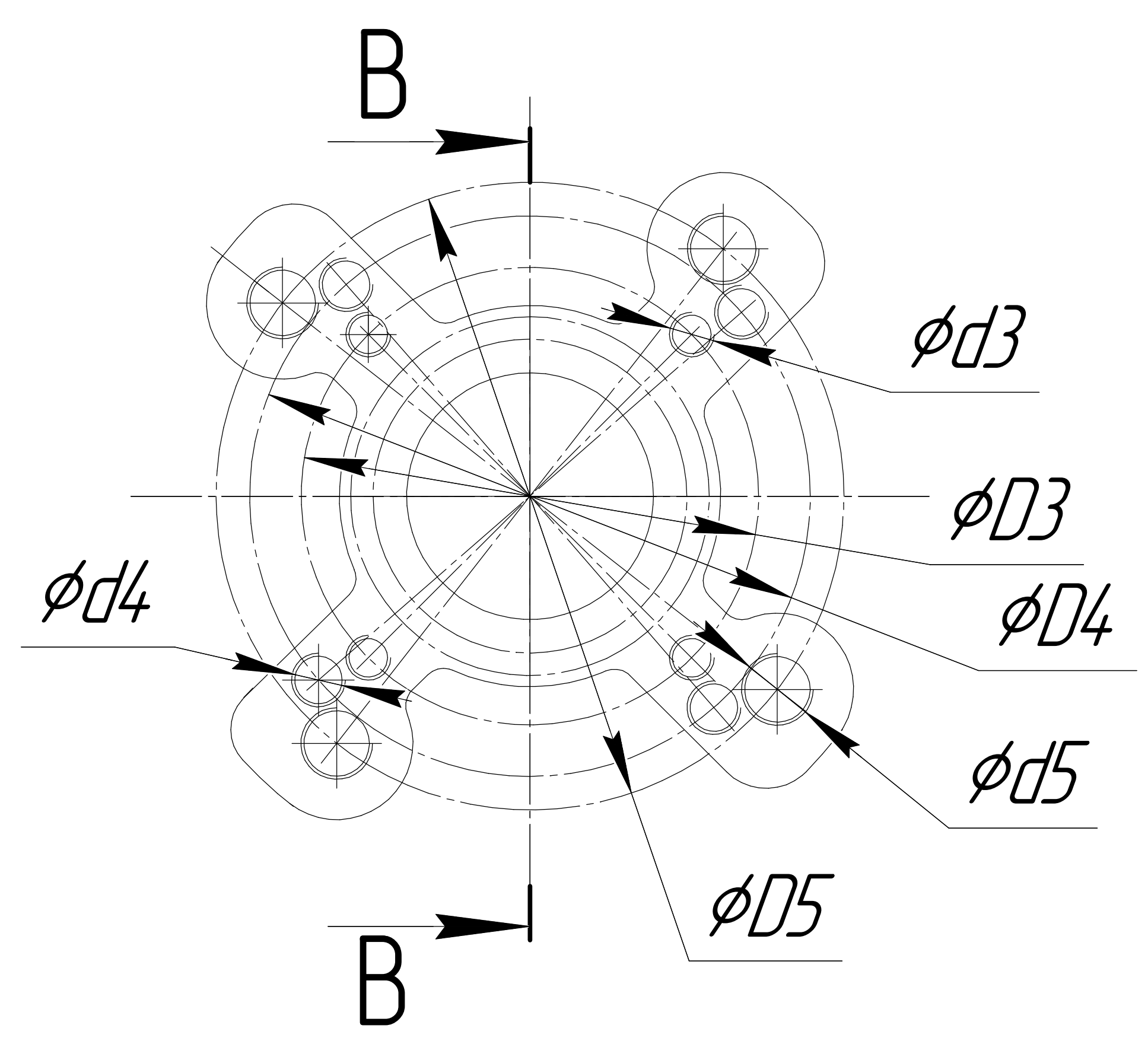
Рисунок А.5 – Механизм М30Ф группы 500 с внутренним присоединением по ISO ГОСТ Р 3427-20137 Остальное см. рис. А.4
