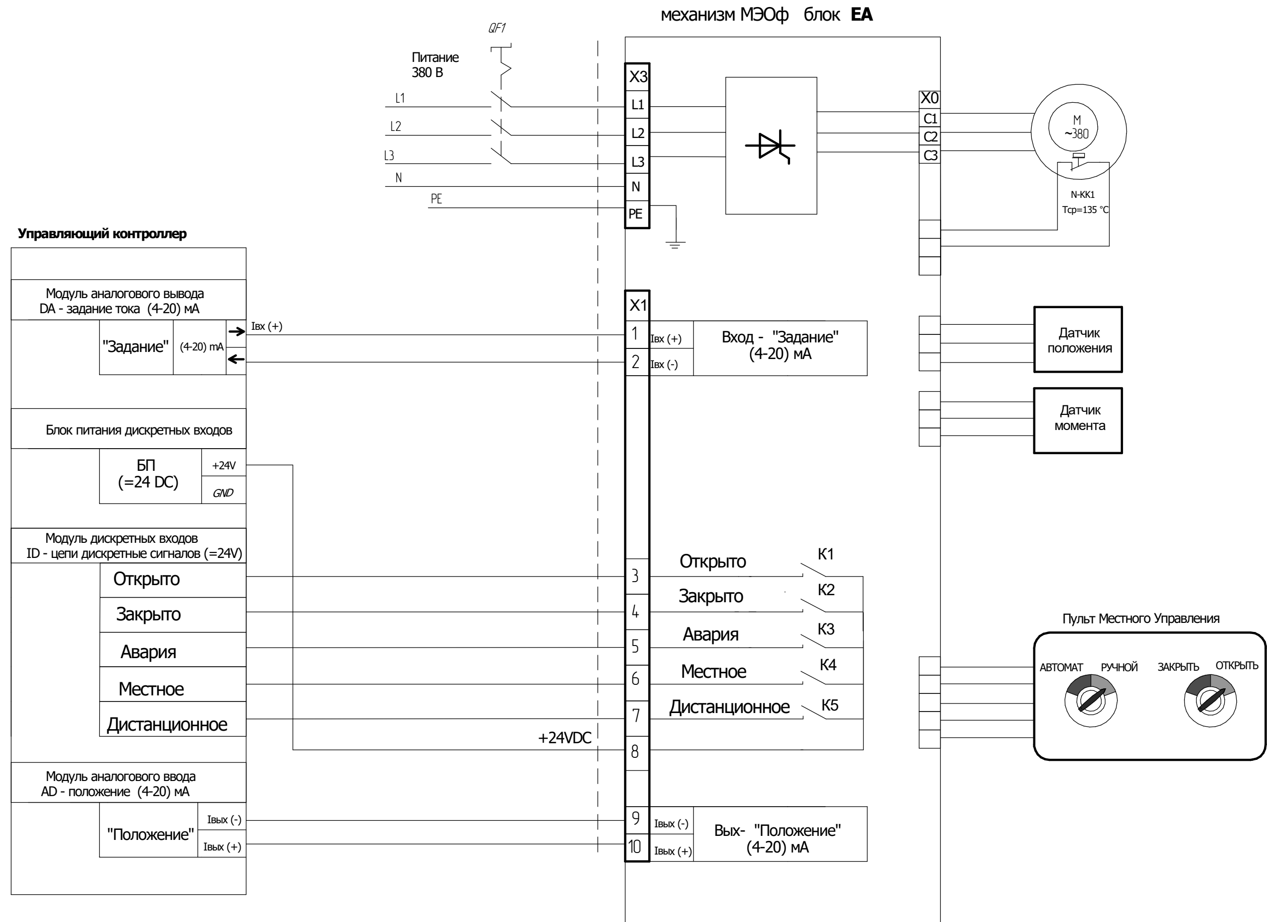
Рисунок В.2 – Схема подключения механизма МЭОФ с блоком ЕА. Питание 380 В (управление – "позиционер" – (4–20) м А, выходные сигналы – 5 реле)
