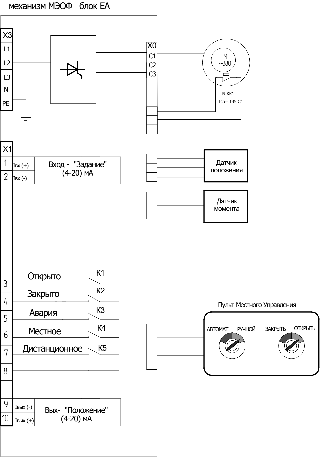
Рисунок Б.2 –Схема электрическая механизма МЭОФ с блоком ЕА. Питание 380 В. (управление – “позиционер” (4–20) мА, выходные сигналы – 5 реле.)
